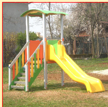
COD MFAL101 H 95 CM Area di Sicurezza - Safety area: cm 715 x 400
