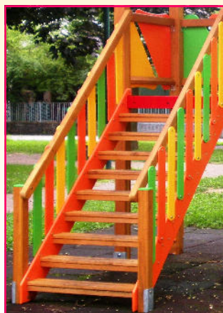
COD MFRIS145-3 Risalita torre - Tower climb H145
