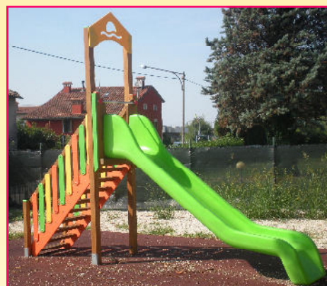
COD MFMT145 H 145 CM Area di Sicurezza - Safety area: cm 370 x 750
