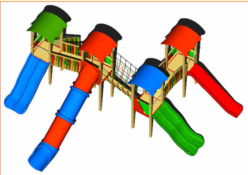
COD MF942 H 145 - 145 - 195 - 145 CM Area di Sicurezza - Safety area: cm 1230 x 1138
