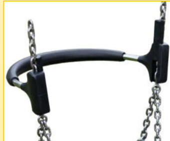
COD MFARC Arco di sicurezza per seg- giolino - Safety arch for child's swing seat
