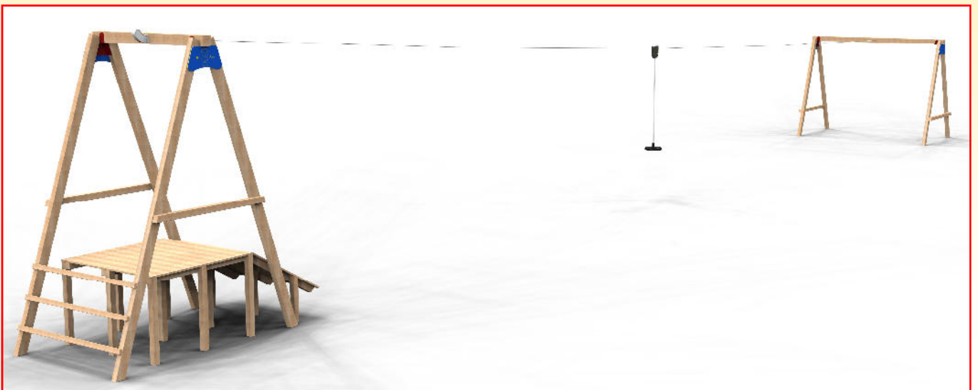
COD MFTE Area di Sicurezza - Safety area: cm 3800 x 400
